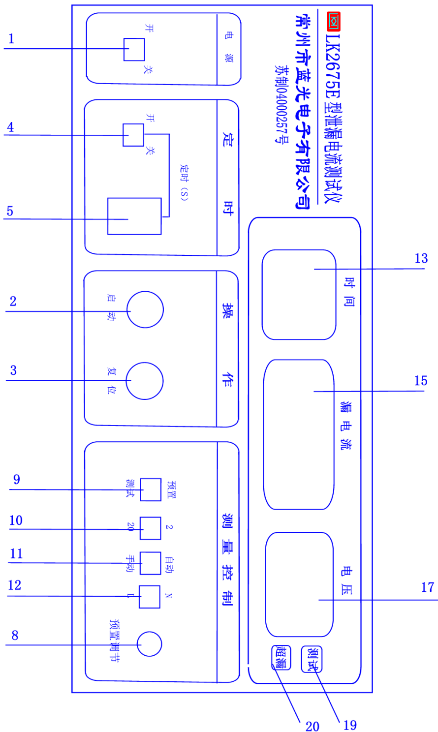
图3 LK2675E型面板示意图
