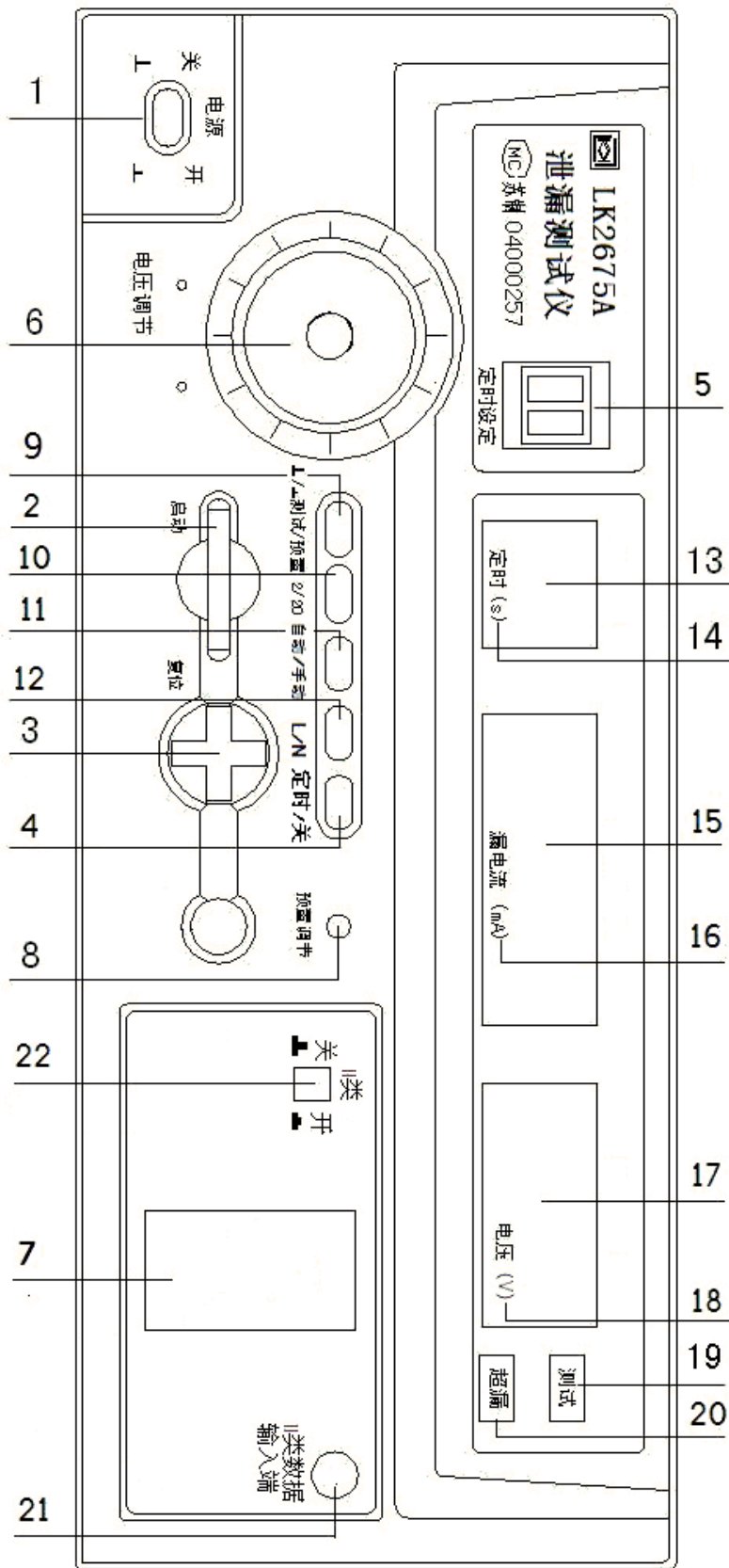
图 2 LK2675A/LK2675B 型面板示意图
