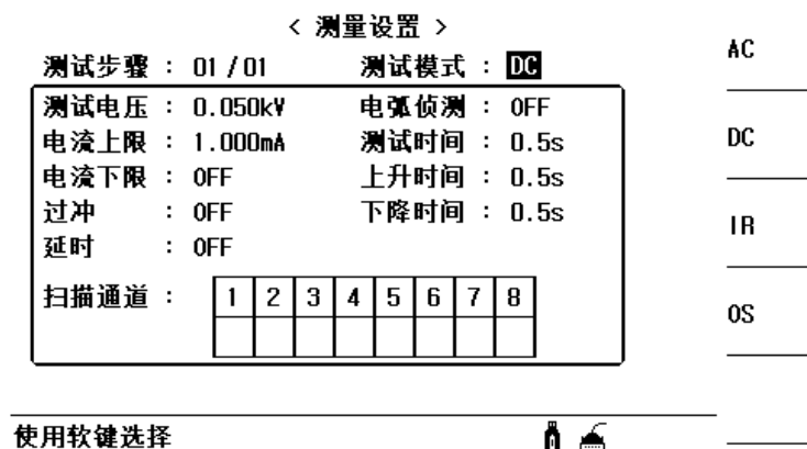
图 4-6 DC 参数设置页面
