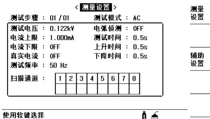
图 4-3 AC 测量设置页面
