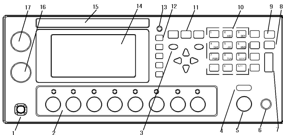
图 3-1 前面板说明
