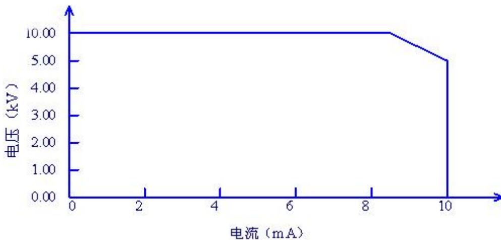
图 3-4 直流电压输出范围
