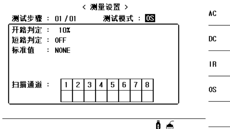
图 4-8 OS 参数设置页面
