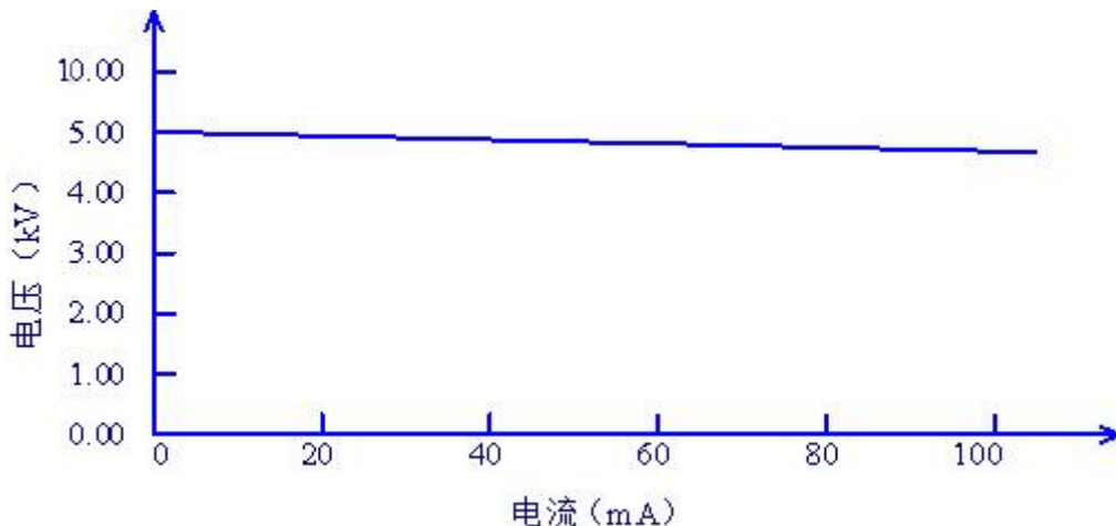
图 3-3 交流电压负载调整率
